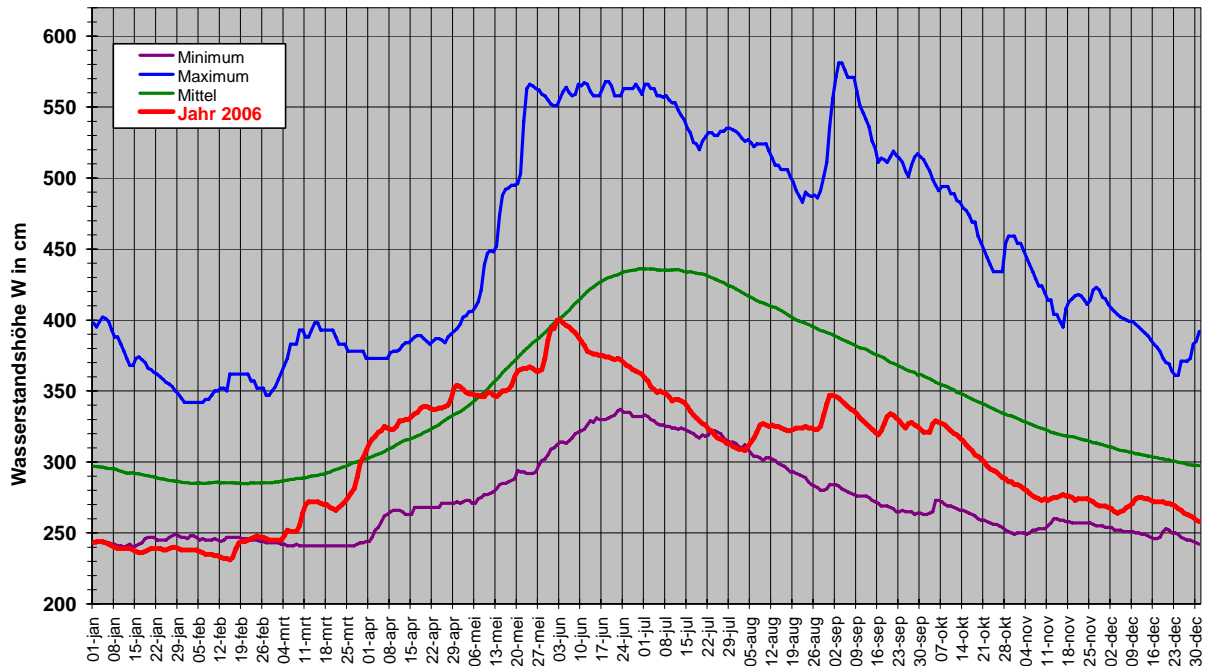
PEGELSTATION BREGENZ - BODENSEE Wasserstandsbewegung von 1864 - 2005 (142 Jahre) - Pegelnullpunkt: 392,14 m ü. Adria
